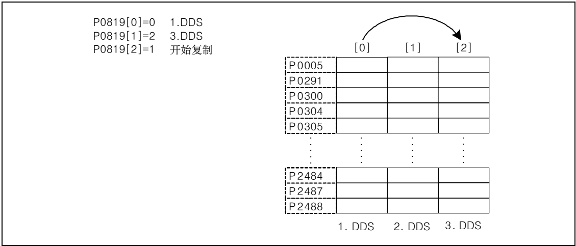
图 3-11 DDS 复制
