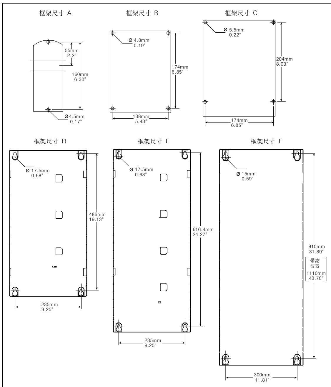
图 2-4 MICROMASTER 440 开孔图
