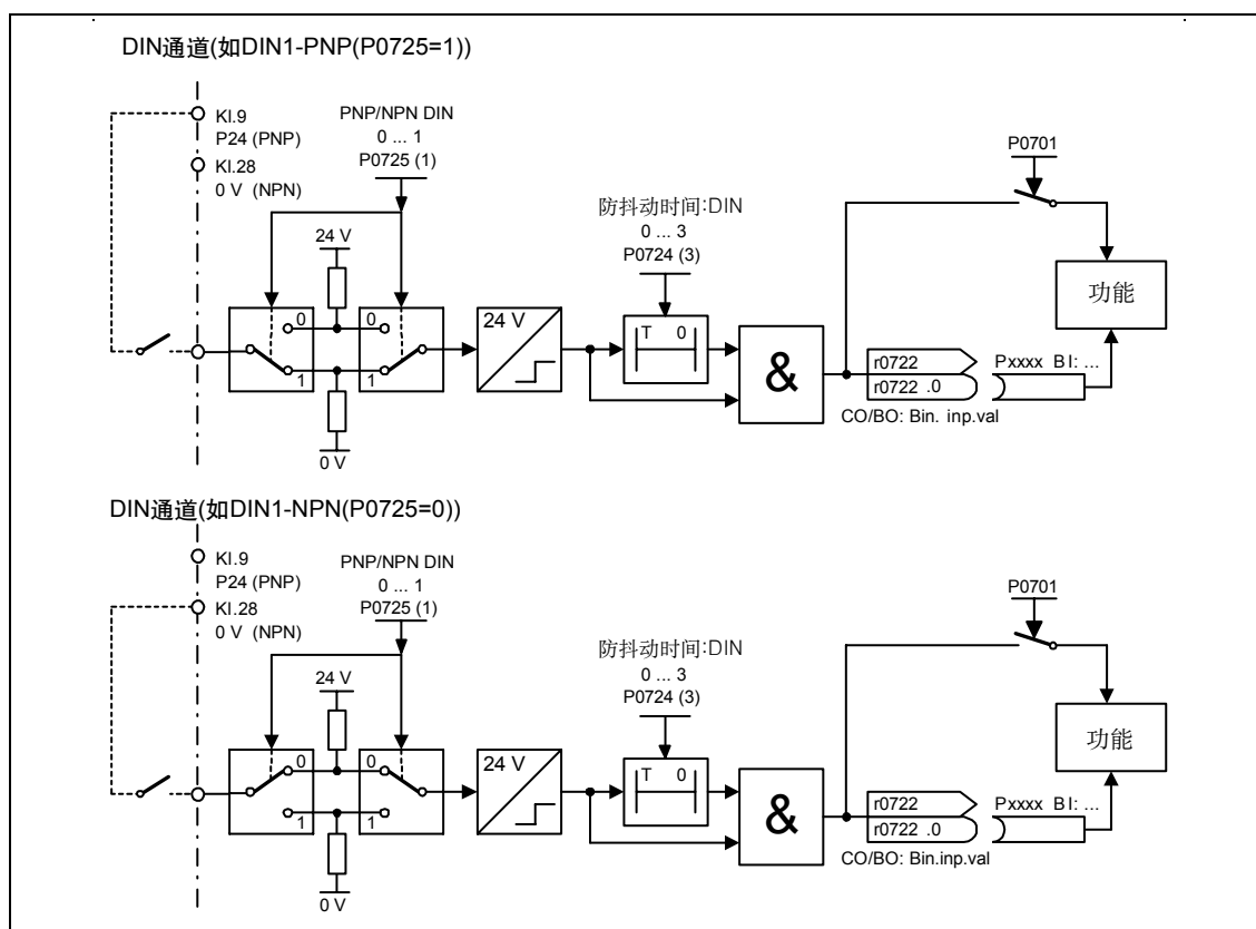
图 3-26 数字量输入
