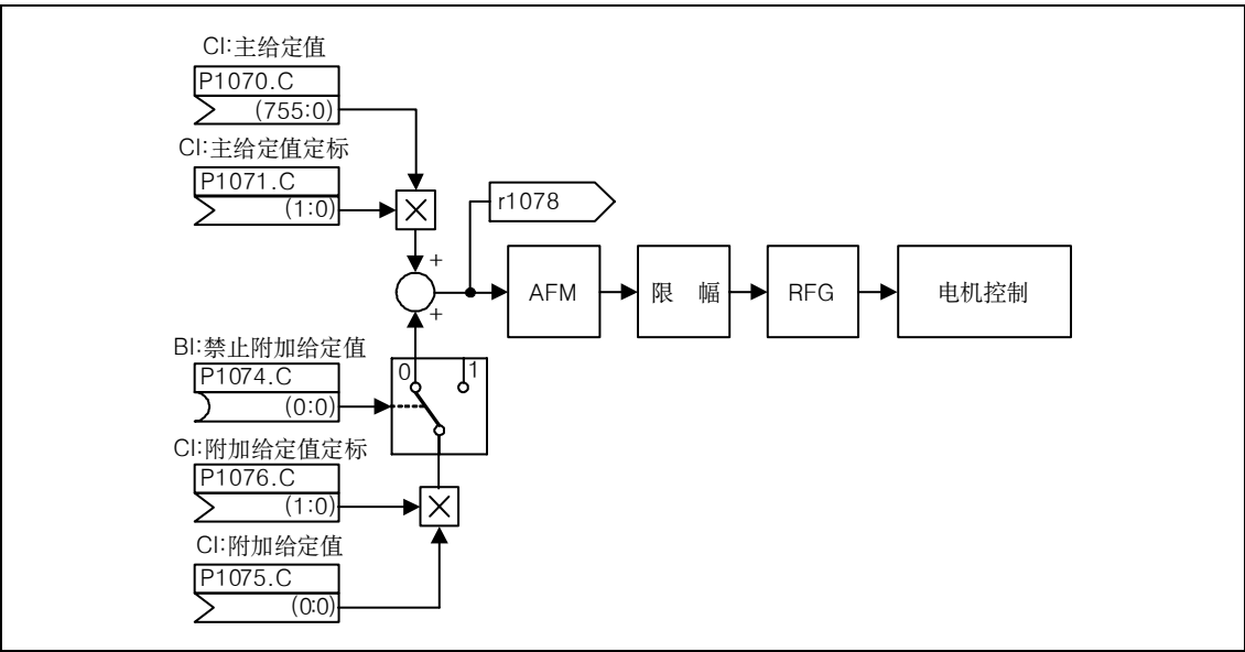
图 3-45 求和
