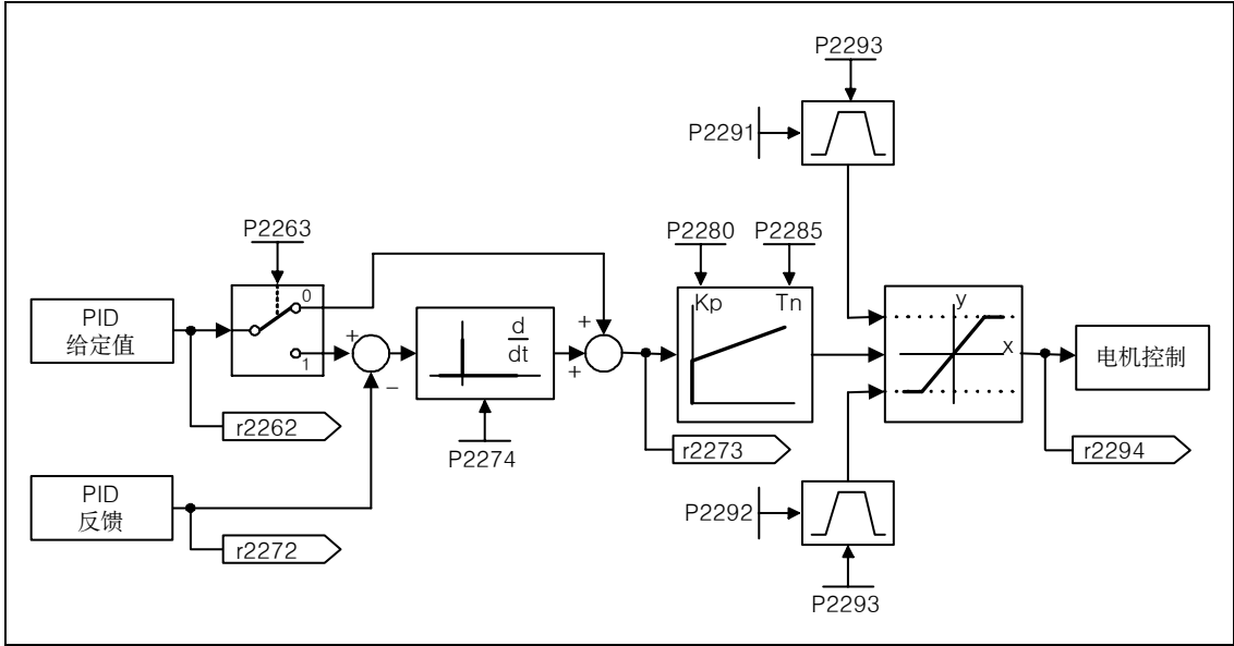
图 3-41 PID 调节器
