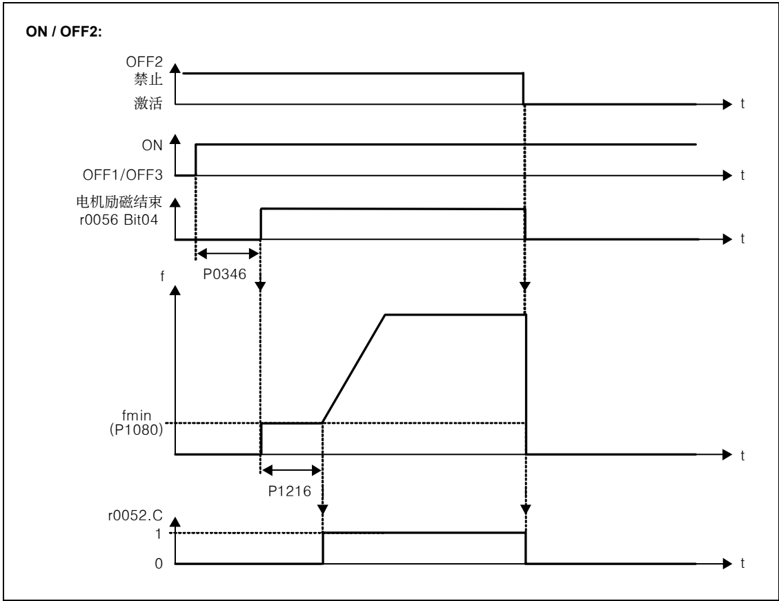
图 3-50 在 OFF2 命令之后的电机停机抱闸
