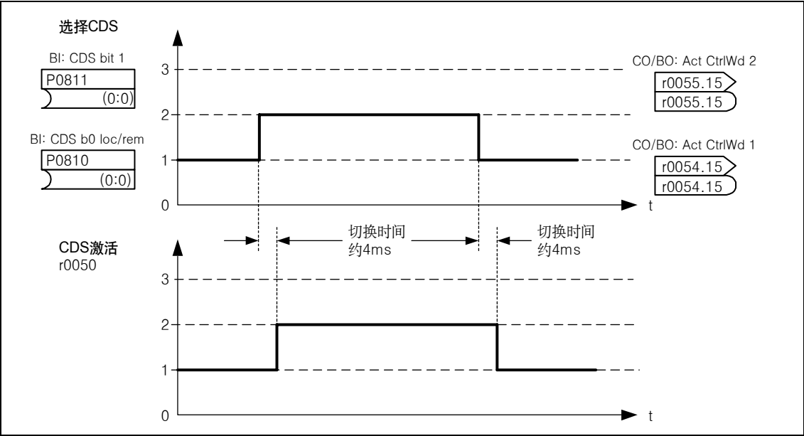
图 3-10 切换 CDS
