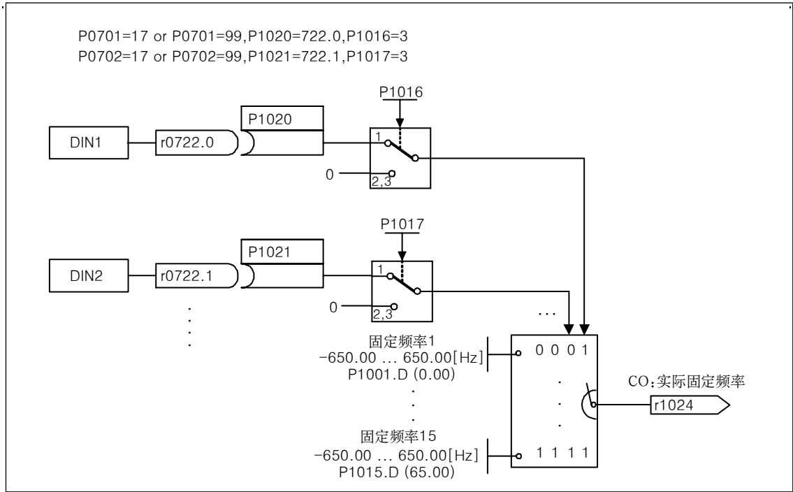
图 3-37 利用二进制码方法，通过 DIN1 选定 FF1、通过 DIN2 选定 FF2 的例子
