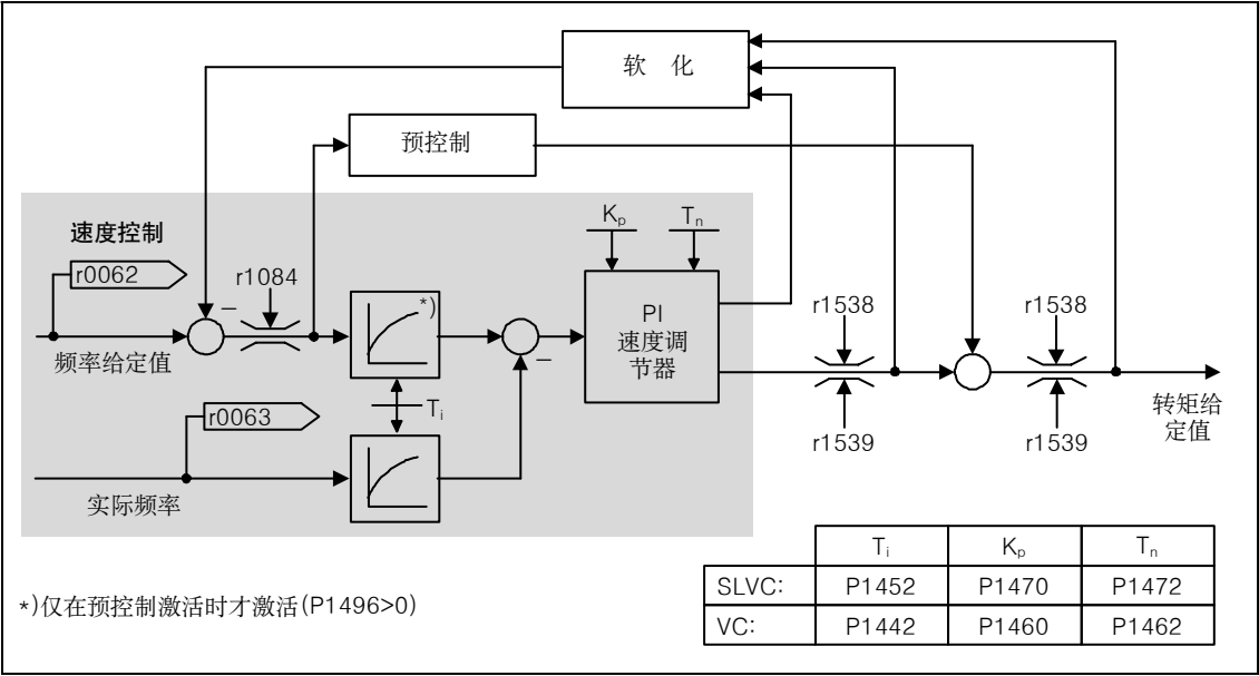
图 3-80 速度调节器
