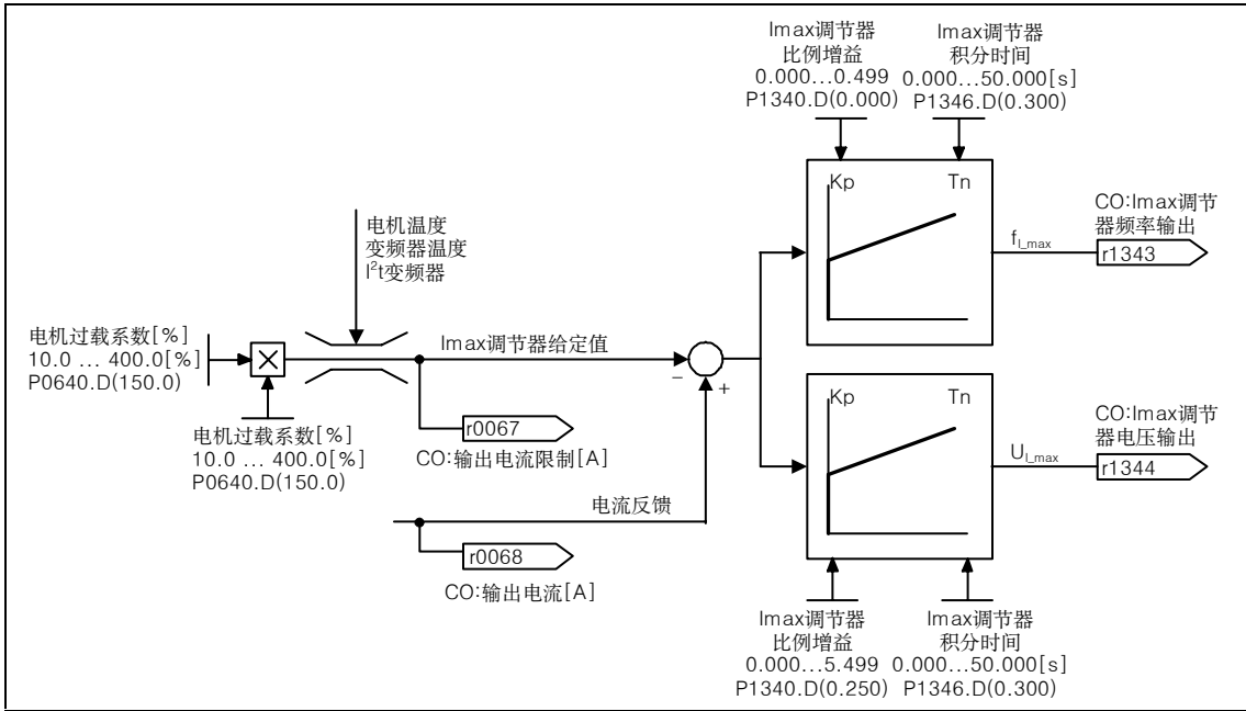
图 3-74 I max 调节器
