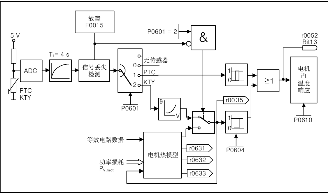
图 3-69 电机热保护
