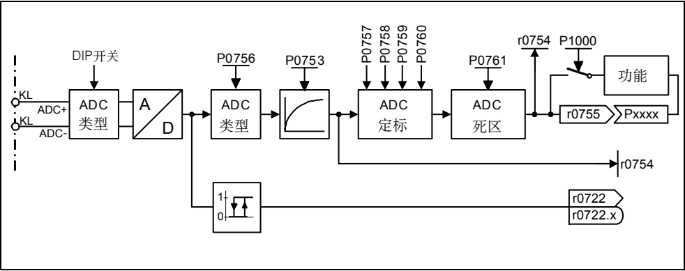
图 3-30 ADC 通道
