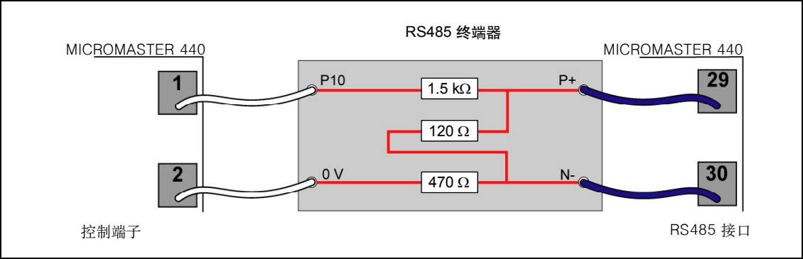
图 3-34 RS485 终端器
