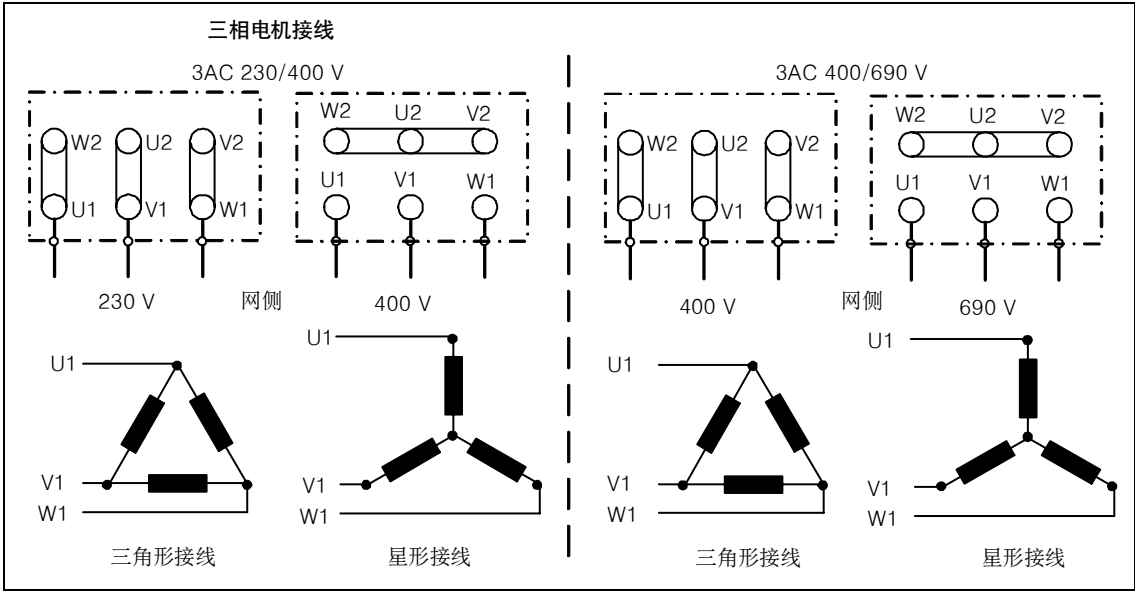
图 3-22 电机端子盒
