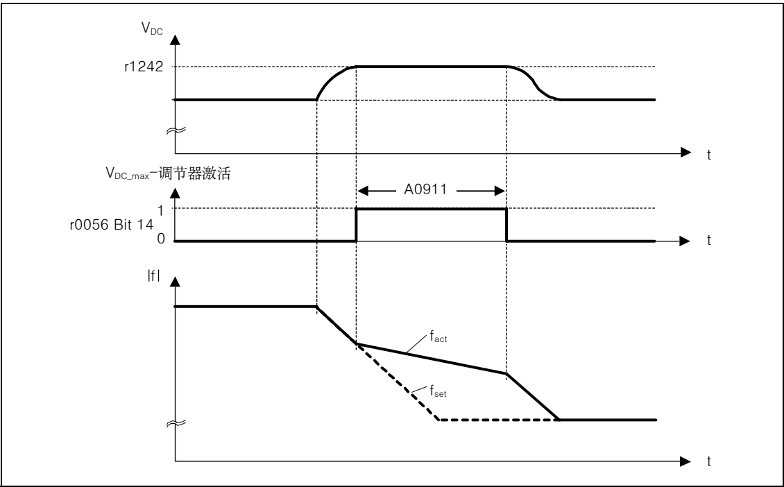
图 3-62 V_{dc-max} 调节器
