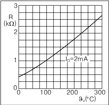
图 3-72 用于 1LG/1LA 电机的 KTY84 特性
