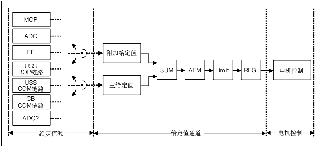
图 3-44 给定值通道
